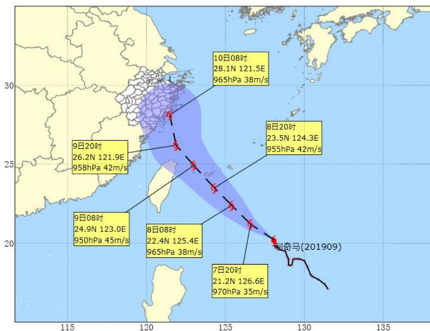
图1 “利奇马” 未来72小时路径概率预报图
